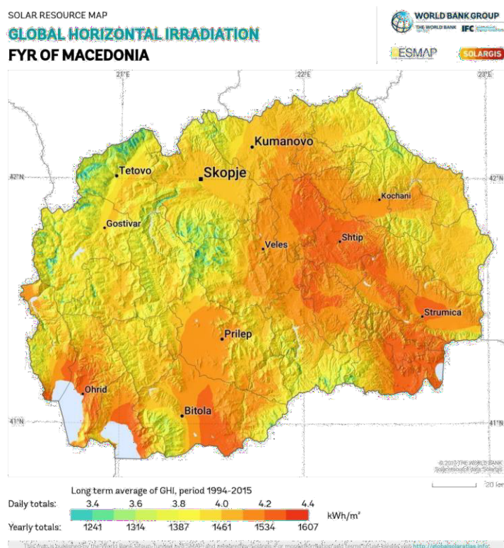
Слика 3. Мапа на годишната просечна ирадијација во \text{kWh/m}^2
